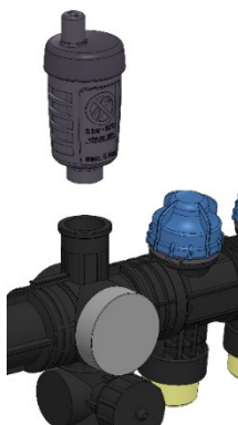
Рисунок 9: Вкручивание воздухоотводчика в пустое соединение
