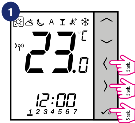
Przytrzymaj przyciski ✓ + < + > przez 5 sekund, aby wejść w tryb instalatora.
