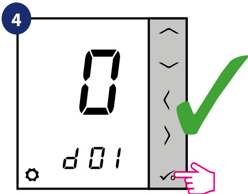
Wybierz parametr przyciskami < lub >. Użyj przycisków ∨ lub ∧ aby zmienić wartość parametru. Wybór potwierdź przyciskiem ✓.
